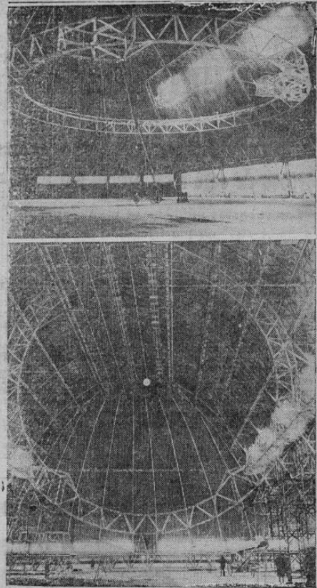
El grabado muestra dos aspectos de los trabajos de construcción del dirigible ZRS-4, que se lleva a cabo en Akron, Ohio, para el gobierno norteamericano
